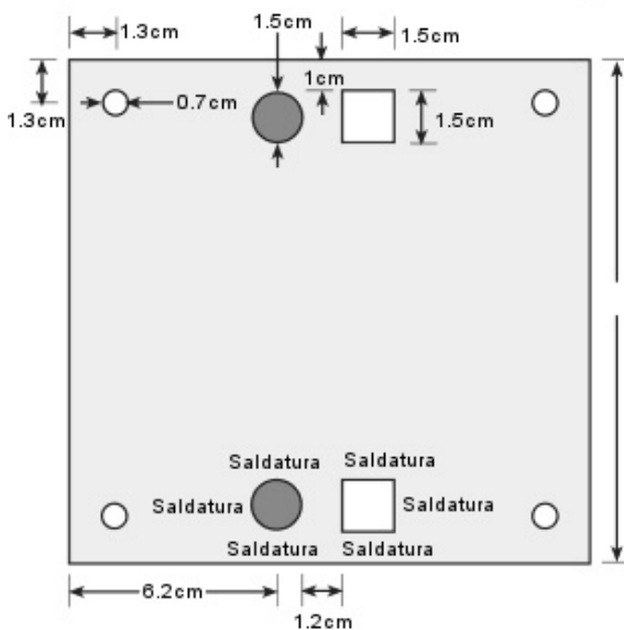
Base del Bersaglio (vista dall'alto)
