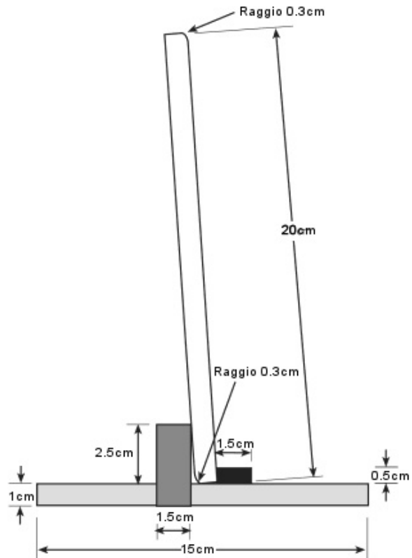
Bersaglio completo Vista laterale
